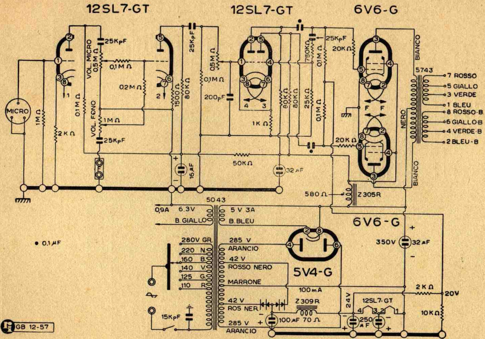
Lo schema elettrico dell'amplificatore mod. G 213-A
